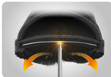
Matrix-Tex™ Lámina PE (1100N) Protección contra clavos y objetos punzantes.
