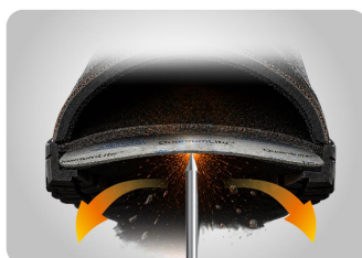
Matrix-Tex™ PE Стелька (1100Н) Сверхлёгкая защита с повышенной гибкостью.
